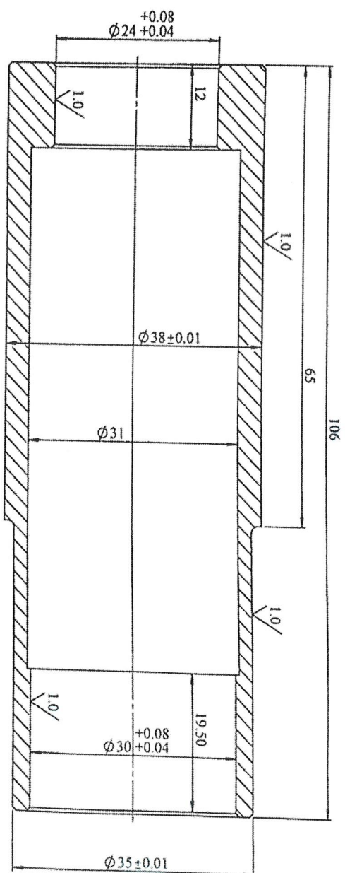
Mặt cái A-A
