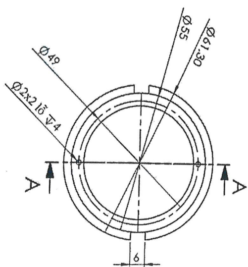
Chi tiết 1
